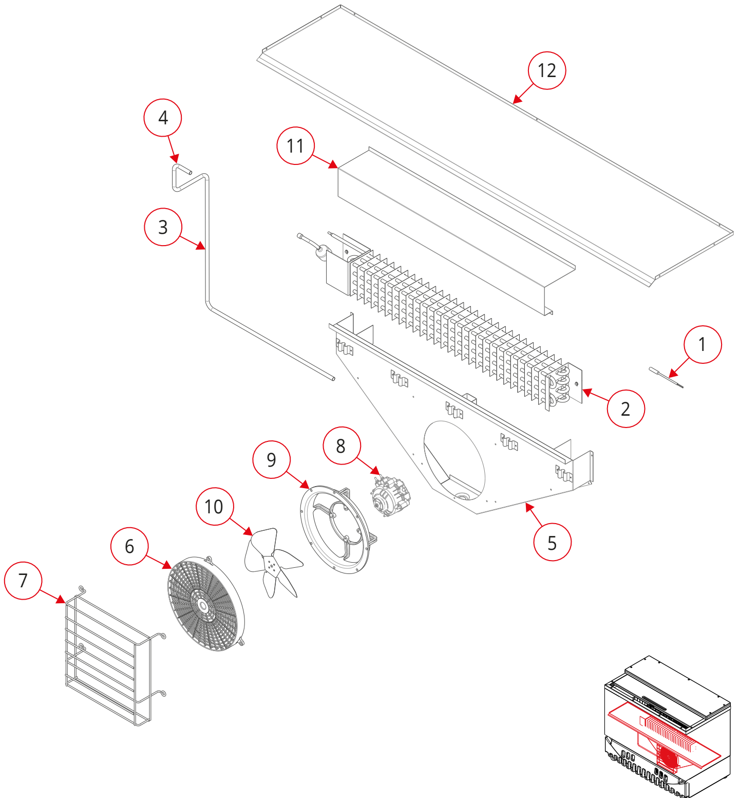
ENSAMBLE EVAPORADOR
