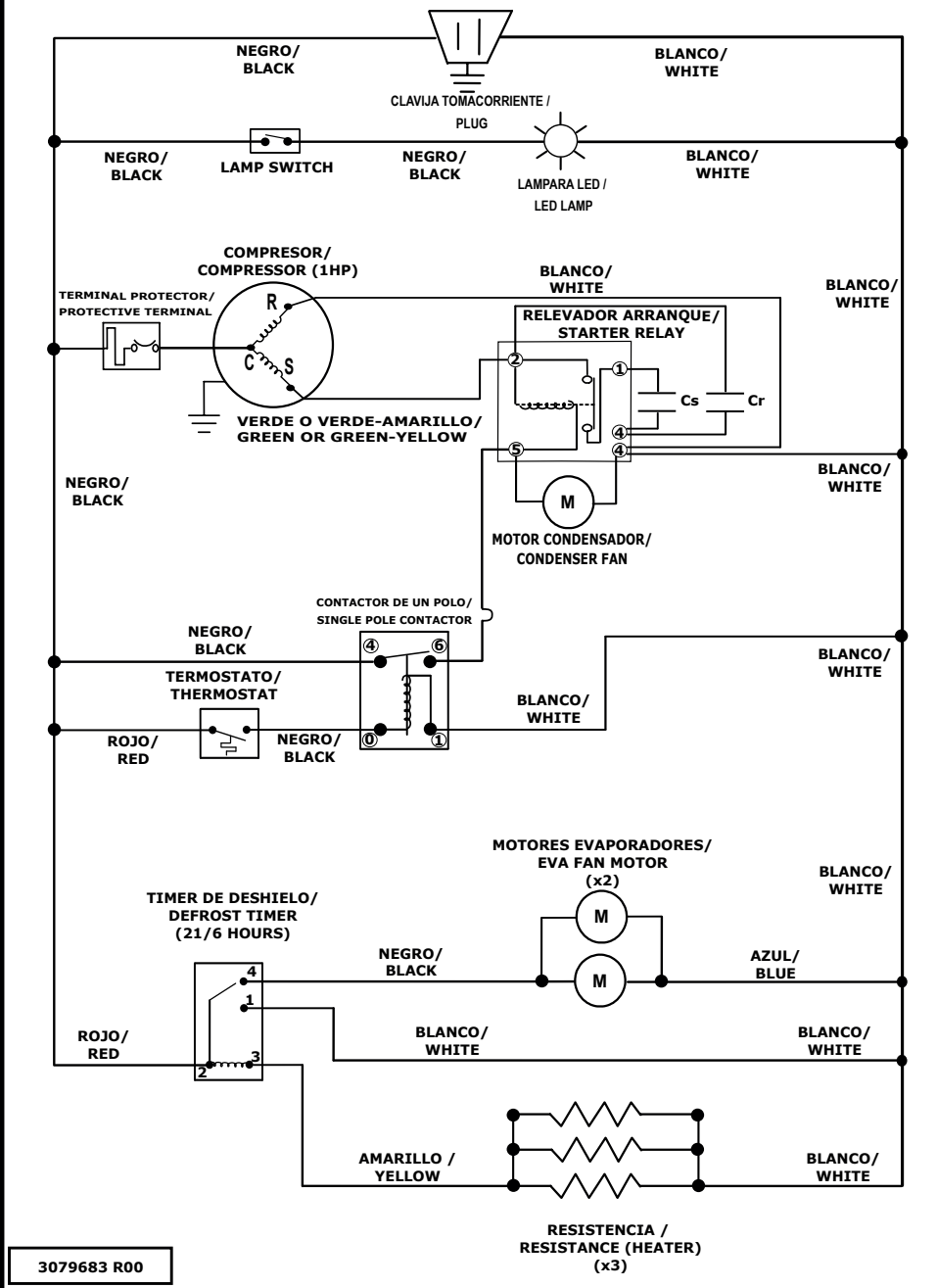
DIAGRAMA ELECTRICO UNIDAD INTEGRAL CONGELACION 220V 60Hz / ELECTRICAL DIAGRAM INTEGRAL UNIT FREEZER 220V 60Hz
