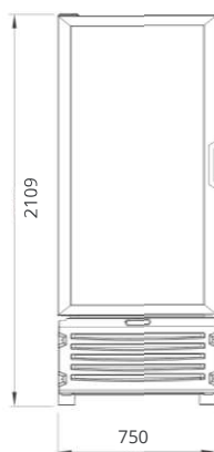
FRENTE
