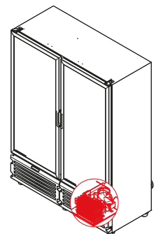
ENSAMBLE CONDENSADOR
