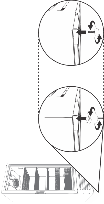
Patín nivelador / Tornillo nivelador
