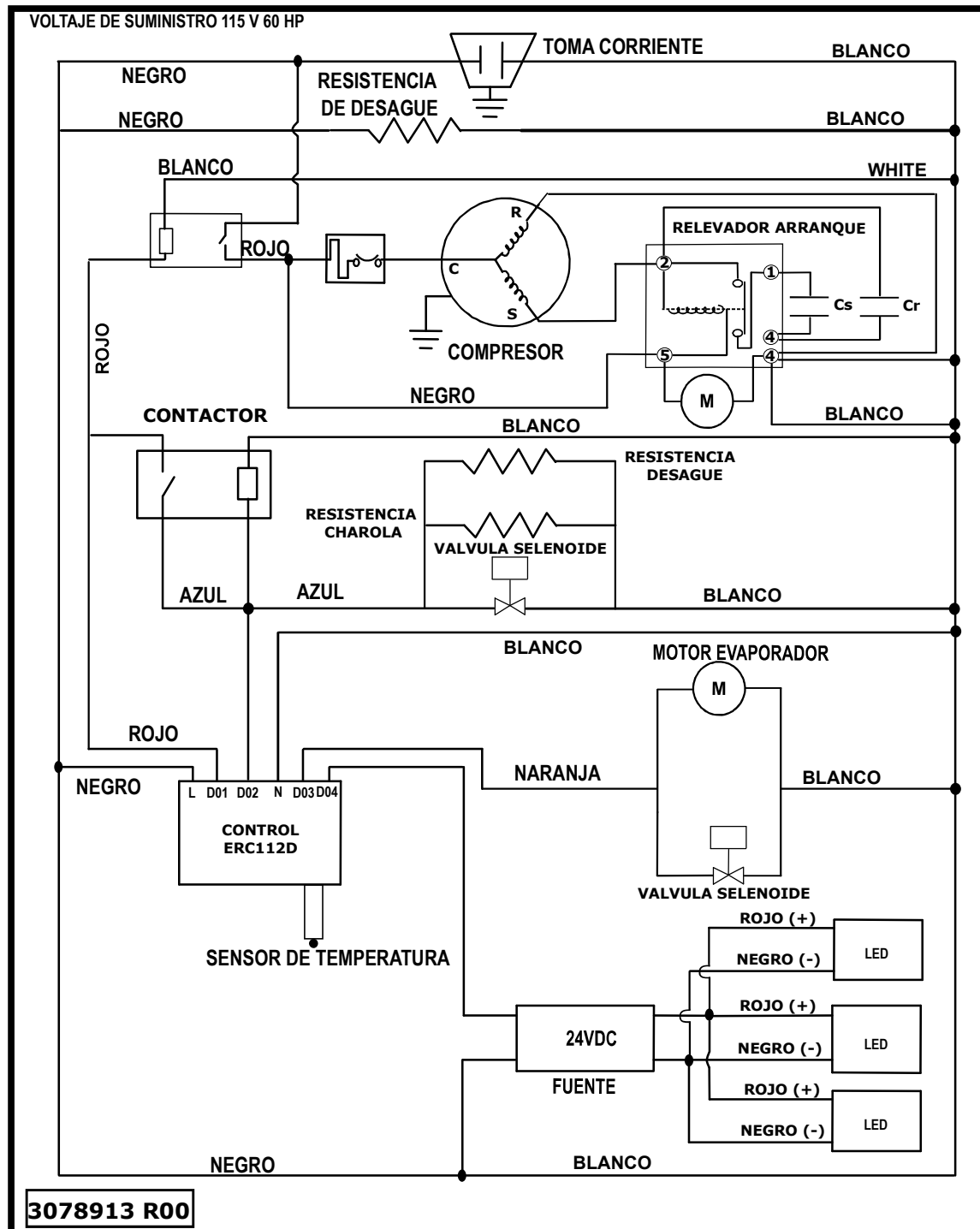
DIAGRAMA ELECTRICO
