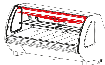
ENSAMBLE EVAPORADOR
