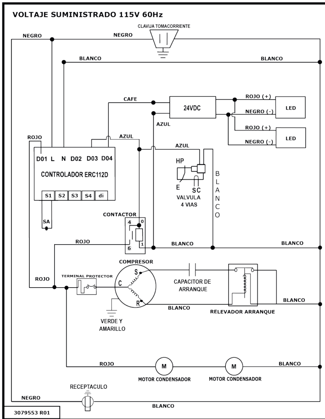
DIAGRAMA ELECTRICO
