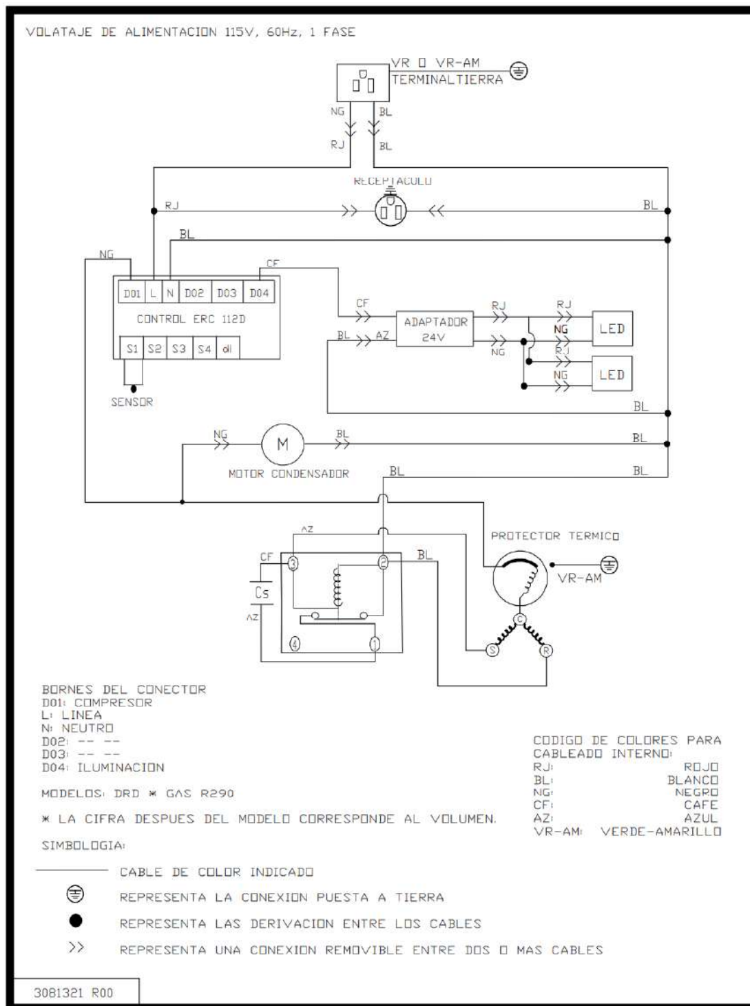
DIAGRAMA ELÉCTRICO
