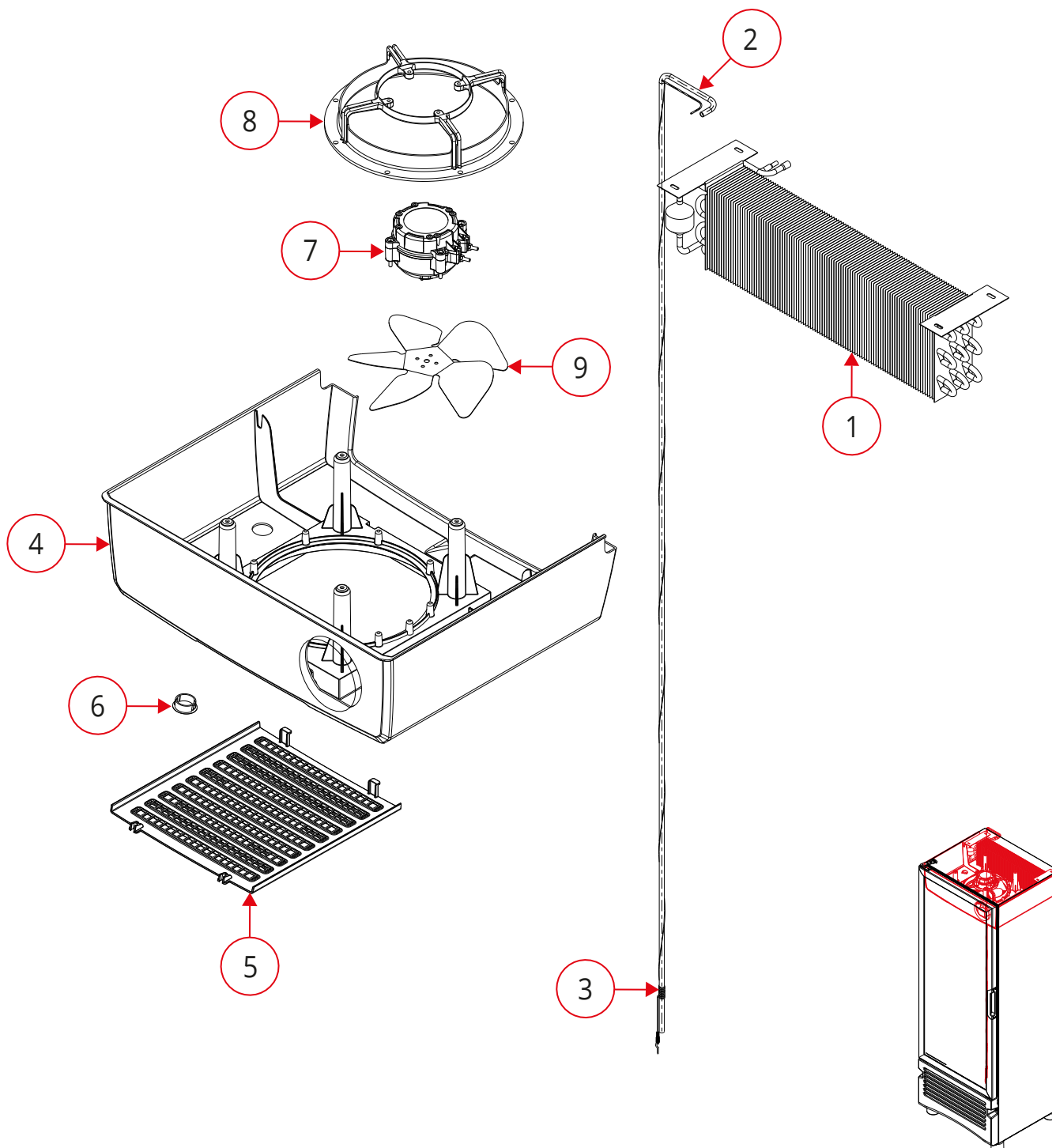
ENSAMBLE EVAPORADOR
