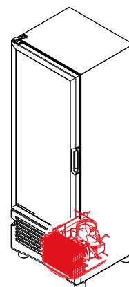
ENSAMBLE CONDENSADOR
