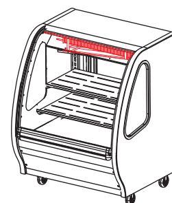
ENSAMBLE EVAPORADOR
