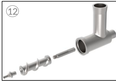
Unidad de Molienda
