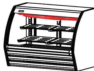
ENSAMBLE EVAPORADOR
