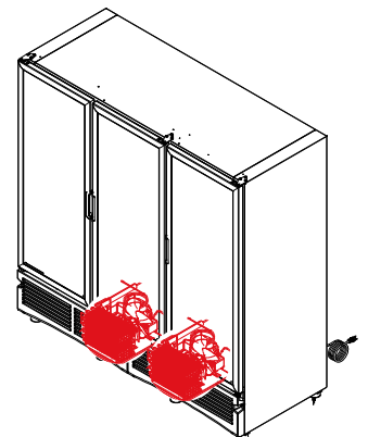
ENSAMBLE CONDENSADOR
