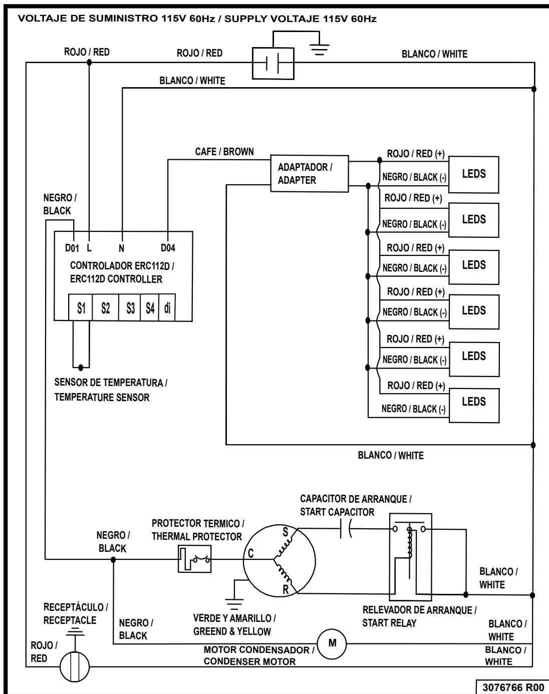
DIAGRAMA ELECTRICO
