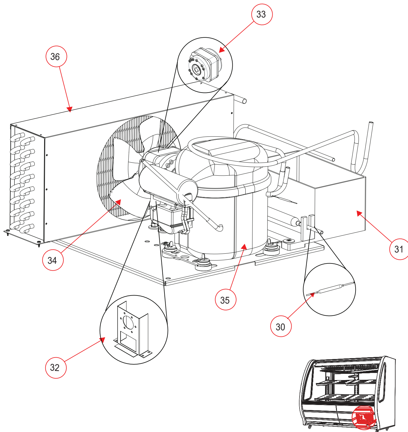
ENSAMBLE CONDENSADOR
